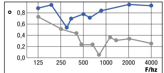
Reflexionsgrad / Degré de réflexion / Degree of reflection
